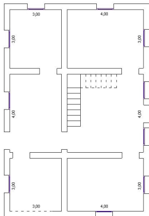
PLANTA BAIXA
